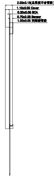
侧视图 横向 10:1
