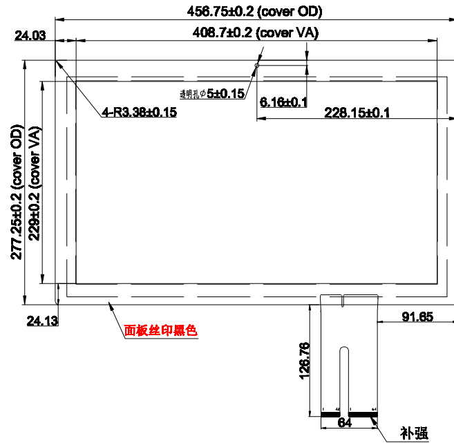
前视图 1:1
