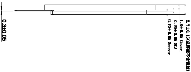
侧视图 横向10:1
